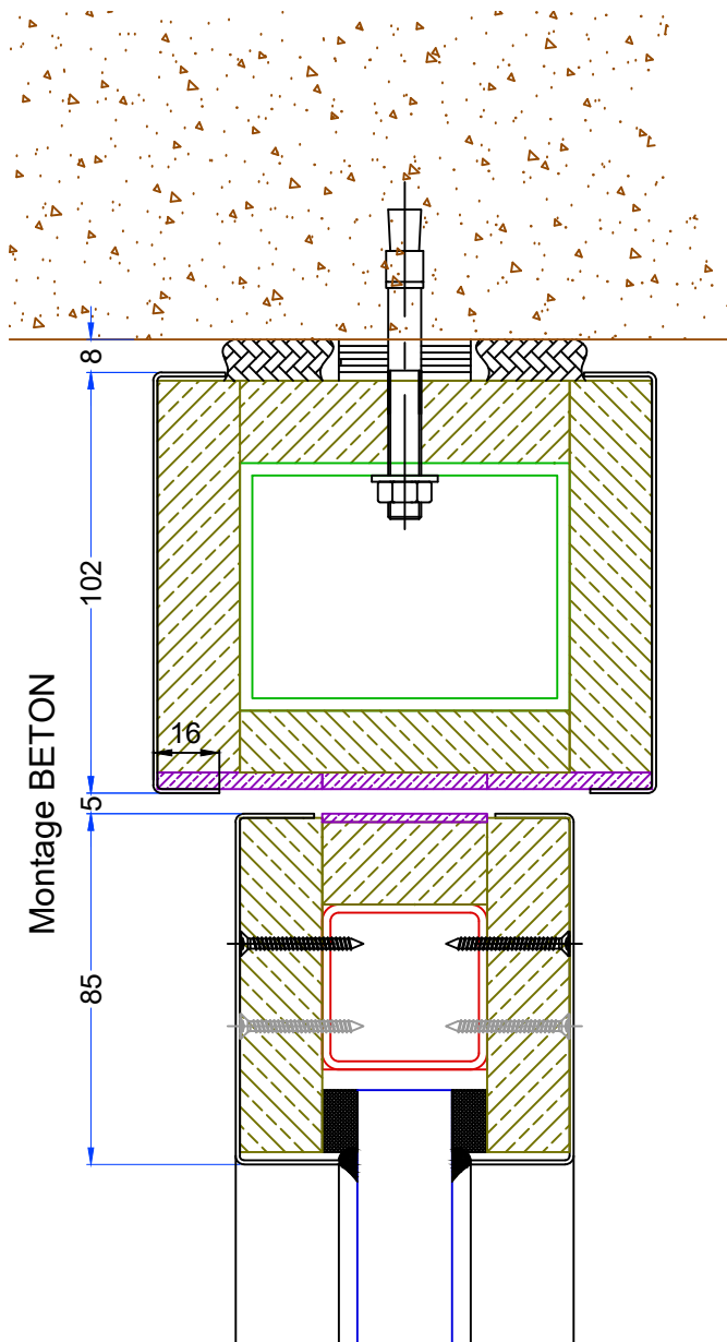
Fixation cheville métal M8
