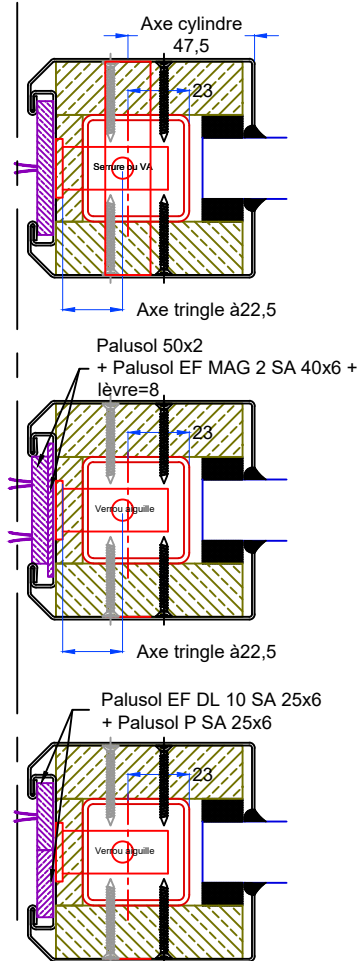
Montage d'une serrure METALUX Réf. 30 & Verrou à aiguille METALUX Réf. 32
