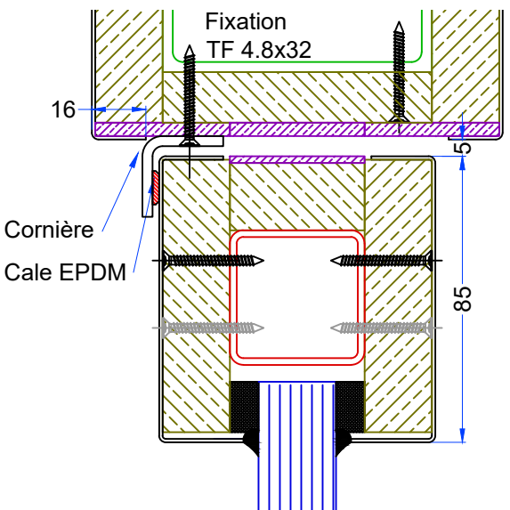
Butée simple action Cornière 27.5x15 lg=65 + cale EPDM
