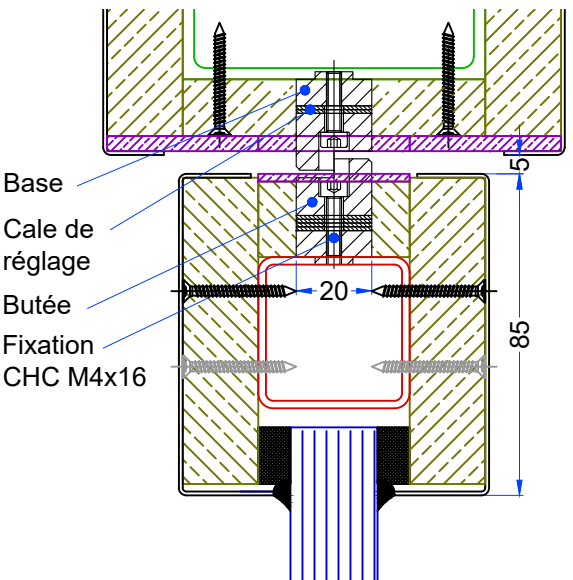
Butée simple action Element réglable Ø20 Base soudée + butée et cale de réglage
