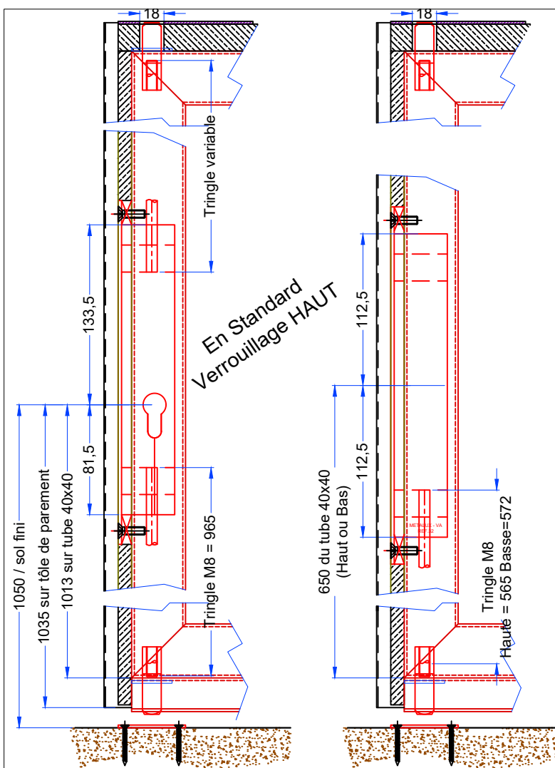
Montage d'une serrure METALUX Réf. 30 & Verrou à aiguille METALUX Réf. 32
