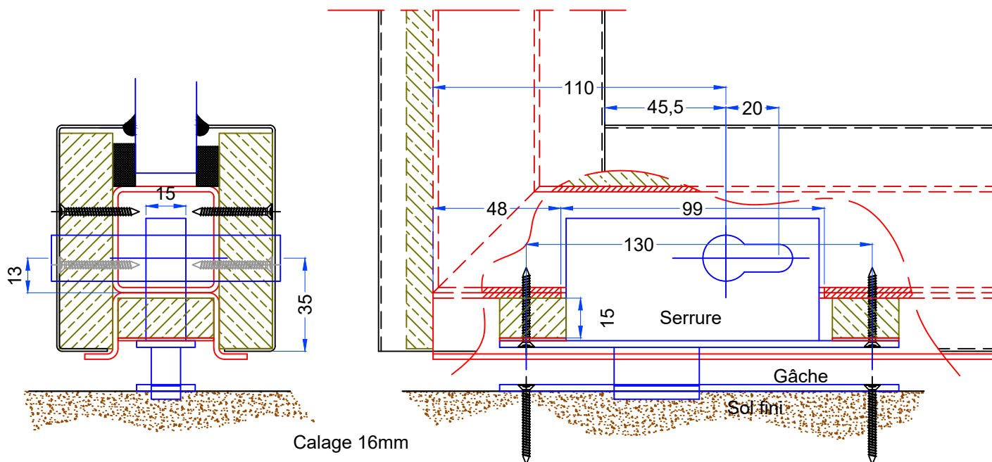
Montage d'une serrure METALUX Réf. 14/46 - Pêne ralongé de 5mm
