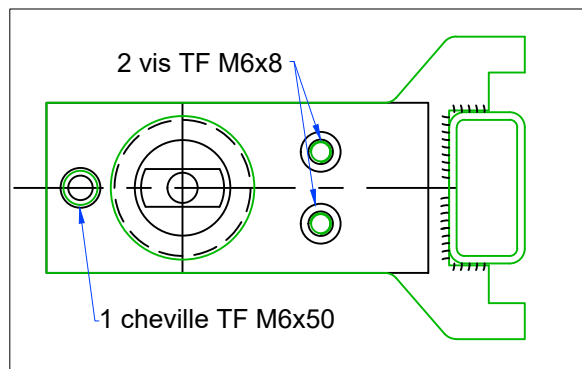
Montage de la crapaudine
