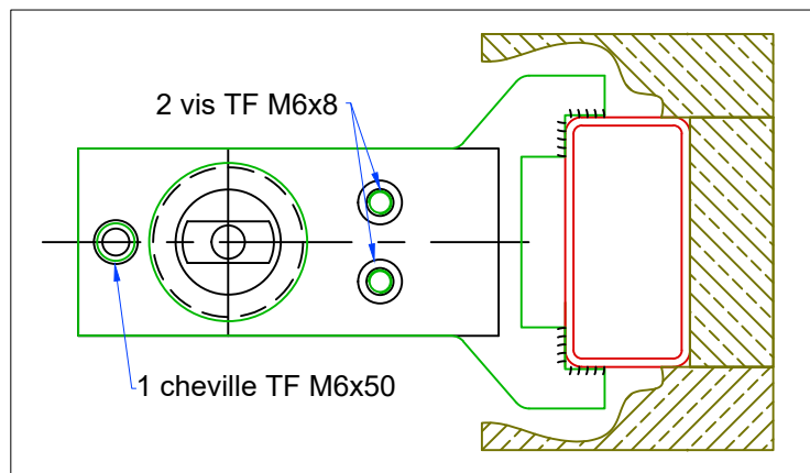
Montage de la crapaudine
