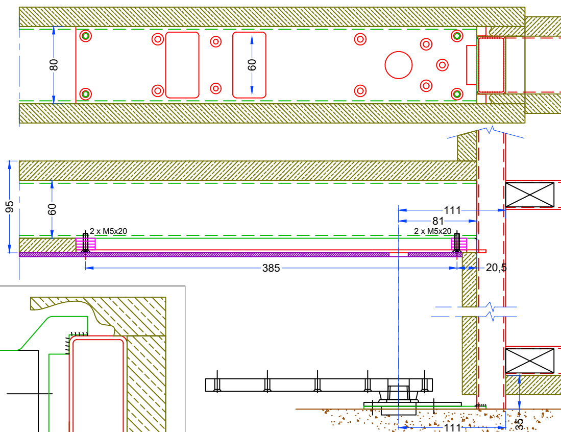
Montage de la crapaudine
