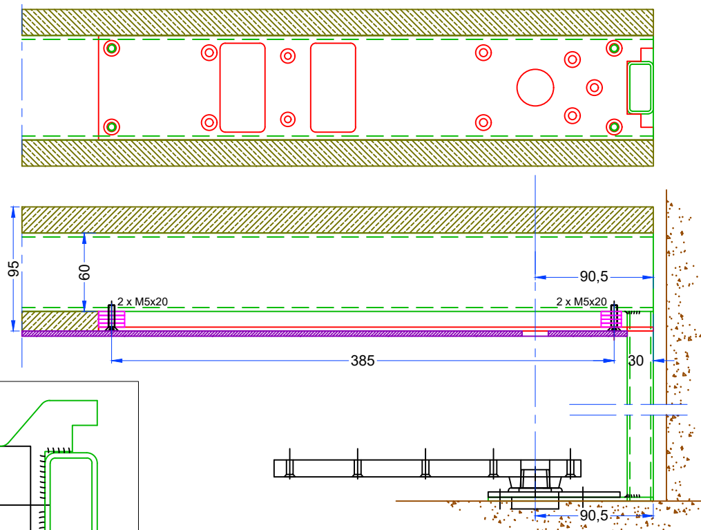
Montage de la crapaudine
