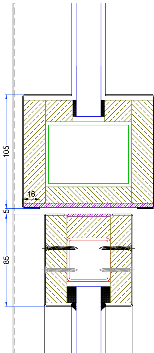
Montage EMV avec imposte vitrée
