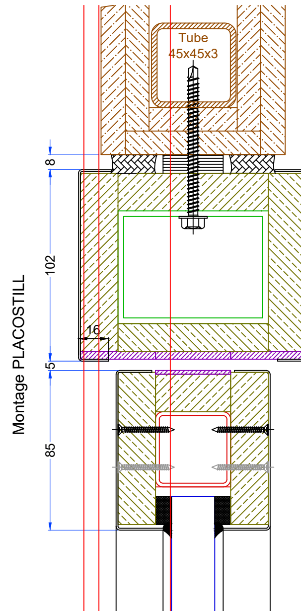
Cloison 98/48 ou similaire Fixation TH 6.3x80
