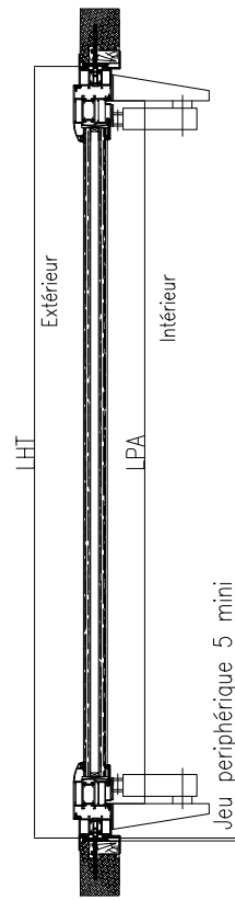
COUPE HORIZONTALE ECH : 1/14
