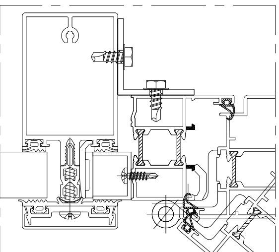
Détail 1 AVEC CHARGE LOURDE Ech : 1/2
