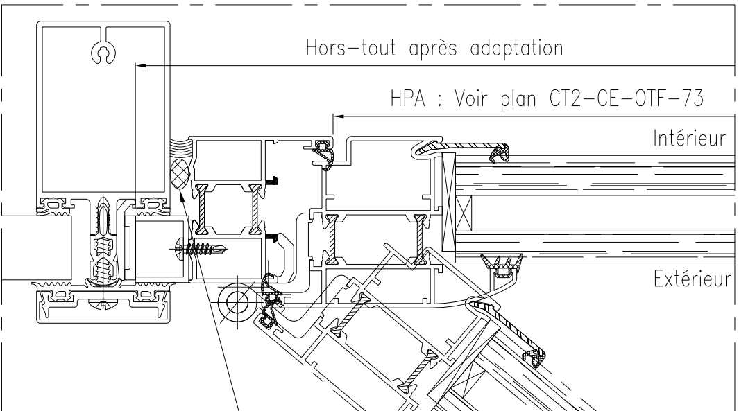
Détail 1 – Ech : 1/2
