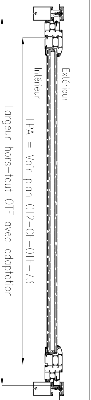
Détail 1 AVEC CHARGE LOURDE Ech : 1/2
