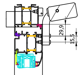
C ( 1 : 4 )
