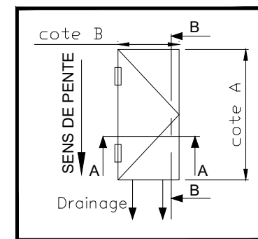
coupe B-B voir plan :CT35-CE-C/LIGHT-29
