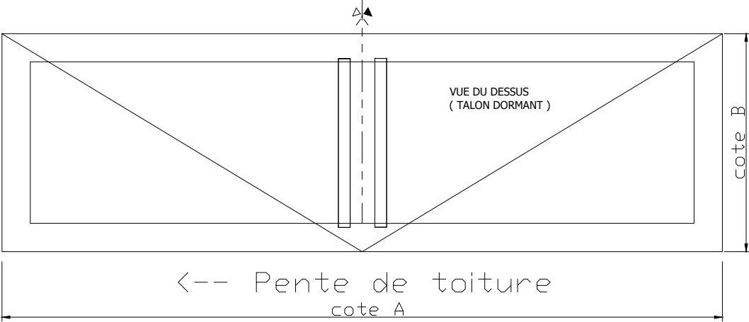
Implantation pour vantail à 1 vérin
