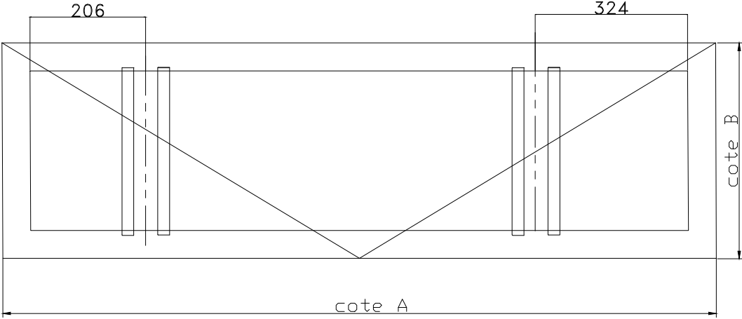
Implantation pour vantail à 2 vérins
