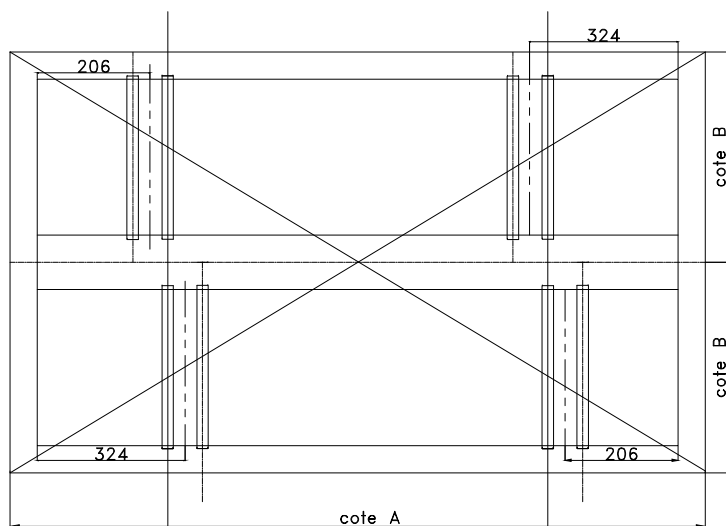
Implantation pour vantail à 2 verins
