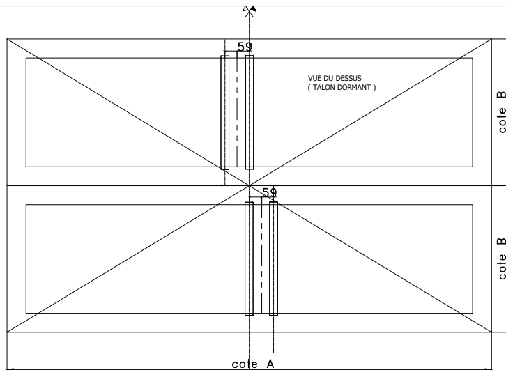
Implantation pour vantail à 1 verin
