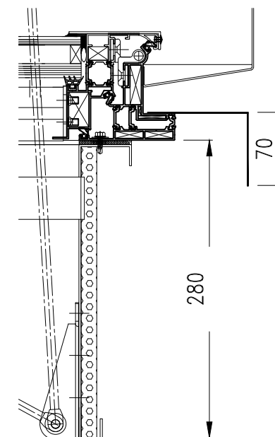
DETAIL COSTIERE
