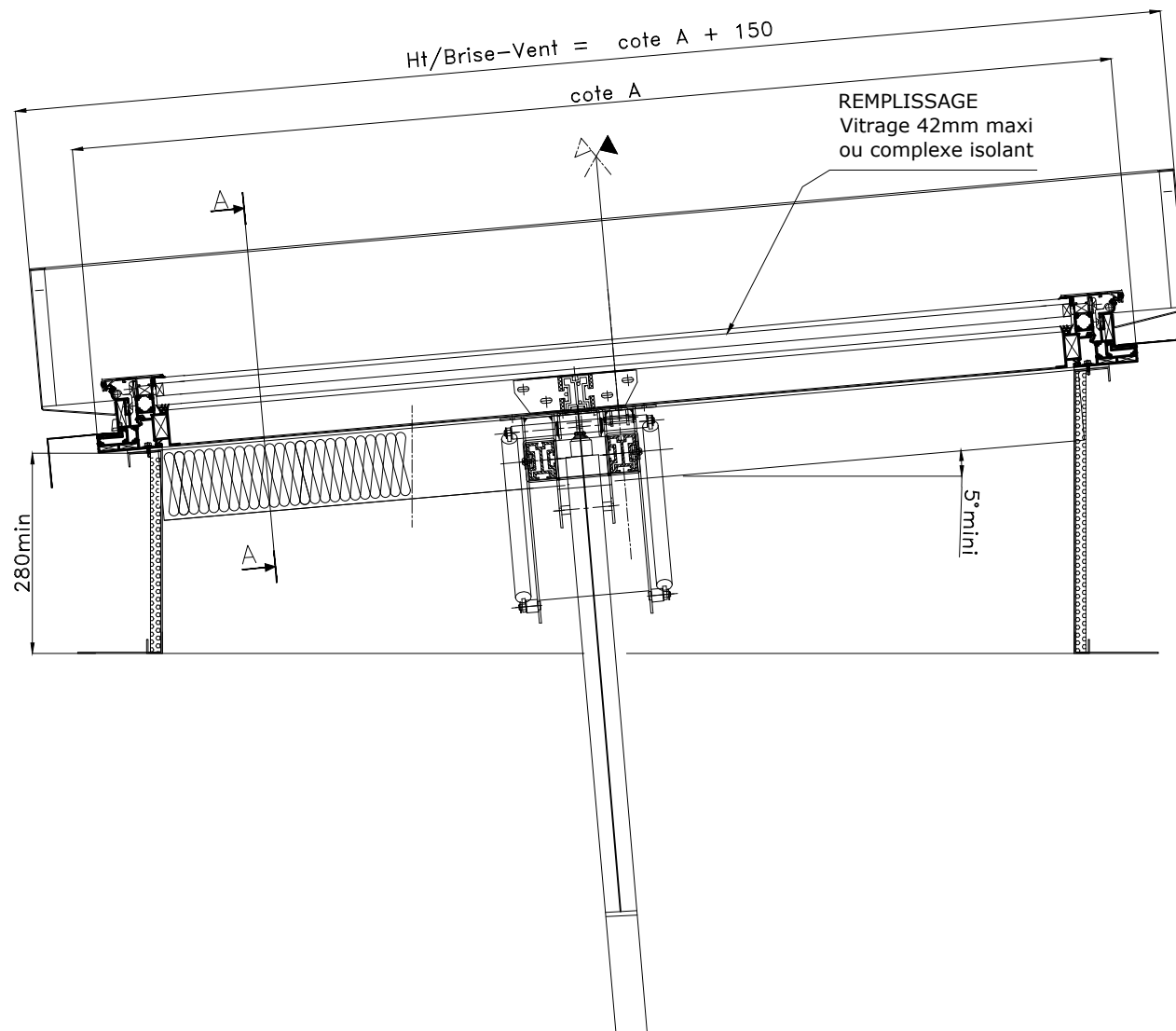
coupe A-A voir plan :CT4-CE-C/LIGHT-07
