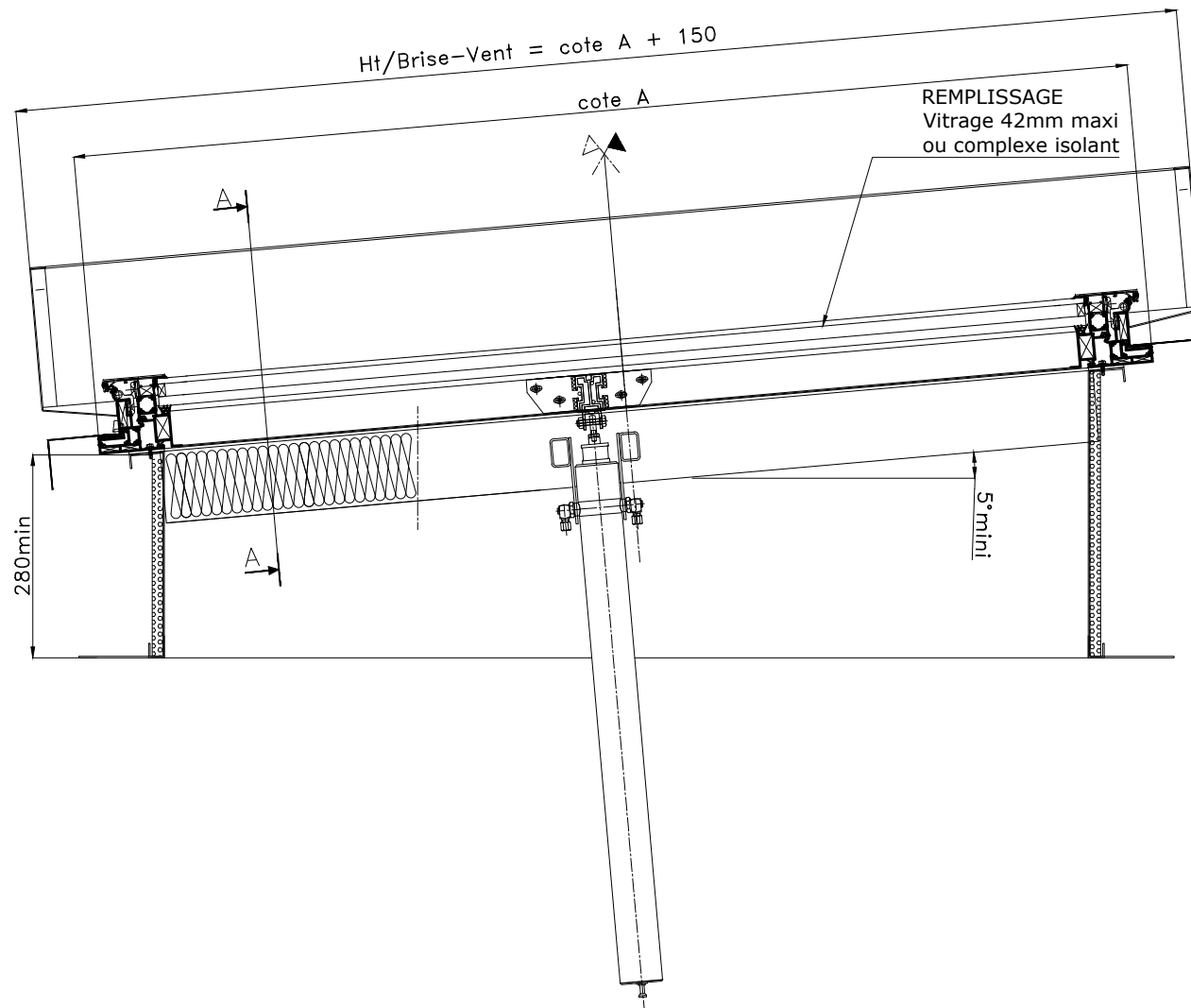
coupe A-A voir plan :CT4-CE-C/LIGHT-07
